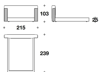
1CO (QUSA) QUEEN USA : LETTO PER MATERASSO / BED FOR MATTRESS 152x205 - 215x239x103H. - H.B.25cm 60x80 2/3 - 84 2/3x94x40 2/3H. - H.B.9 3/4"
