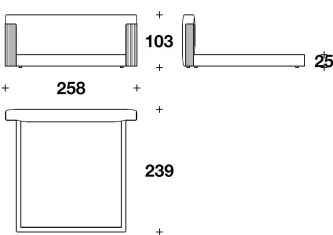
1CO (KUSA) KING USA : LETTO PER MATERASSO / BED FOR MATTRESS 195x205 - 258x239x103H. - H.B.25cm 76 2/3x80 2/3 - 101 2/3x94x40 2/3H. - H.B.9 3/4"
